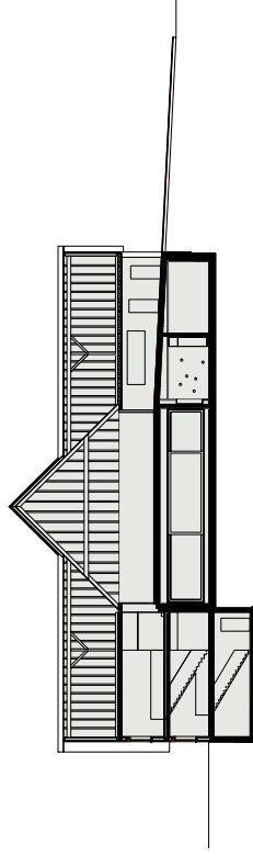
COUPE 1 / SCHNITT 1
