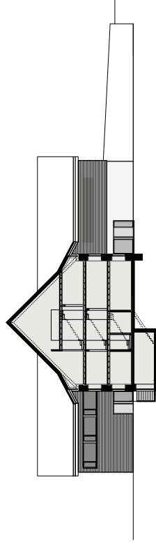
COUPE 3 / SCHNITT 3
